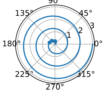
markevery=[16, 24, 30]
