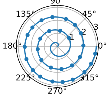
markevery=(0.45, 0.1)
