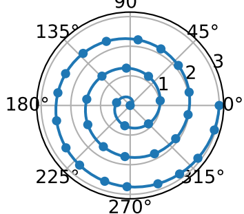
markevery=(0.0, 0.1)
