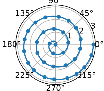
markevery=0.1
