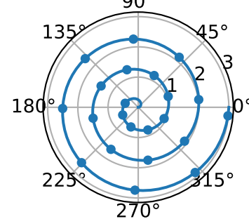
markevery=slice(100, 200, 3)
