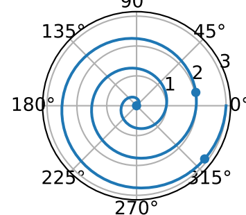
markevery=1.5
